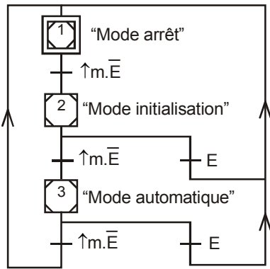
Grafset de fonctionnement global
